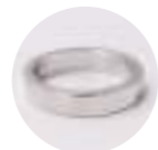
外径23mm 内径19mm 幅4×厚さ2mm
